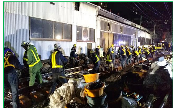
分岐器重軌条化工事
